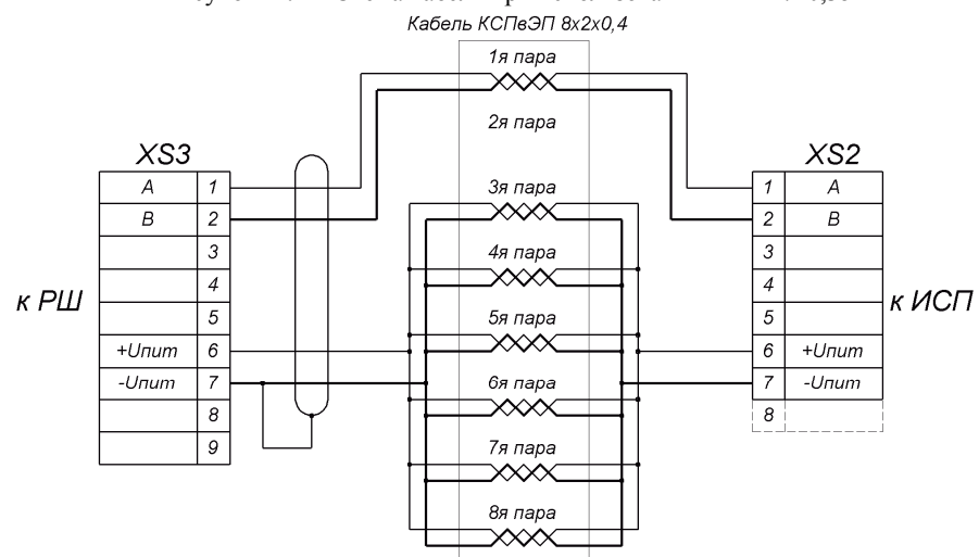
Рисунок М.2 – Схема кабеля при использовании КСПвЭП 8x2x0,4
