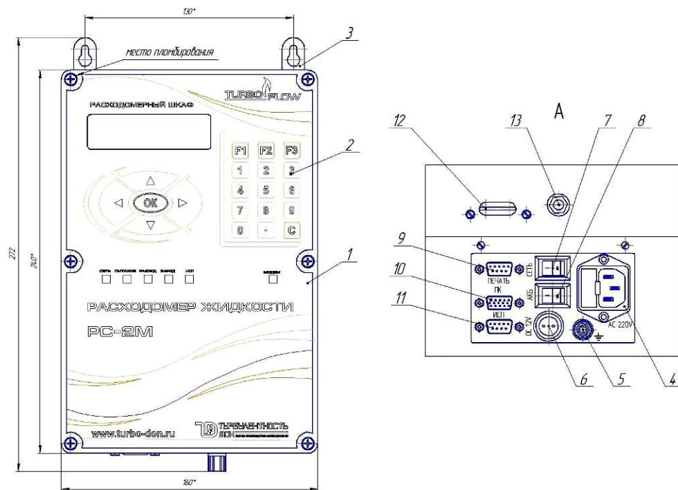
Рисунок В.1 – Внешний вид расходомерного шкафа для одноканального расходомера
