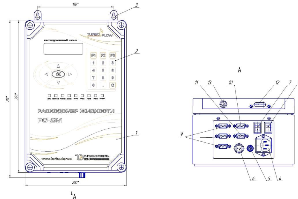
Рисунок В.2 – Внешний вид расходомерного шкафа для многоканального расходомера
