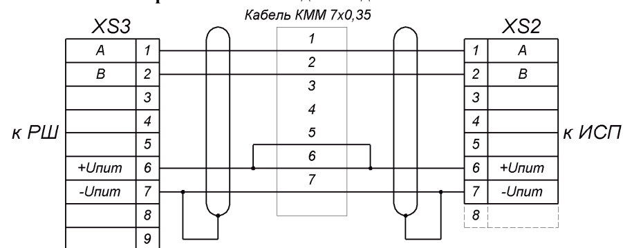
Рисунок М.1 – Схема кабеля при использовании КММ 7х0,35
