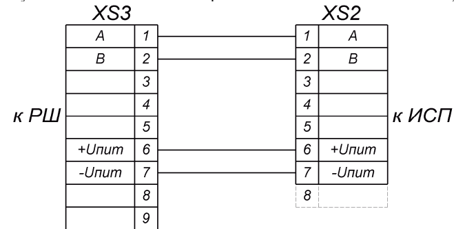
Рисунок М.3 – Проверочный системный кабель
